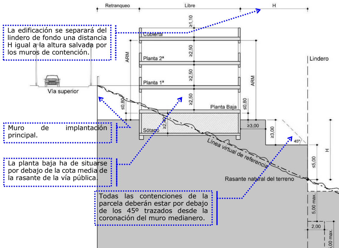
Sección característica de la edificación ladera abajo con pendientes entre 35% y el 50%
