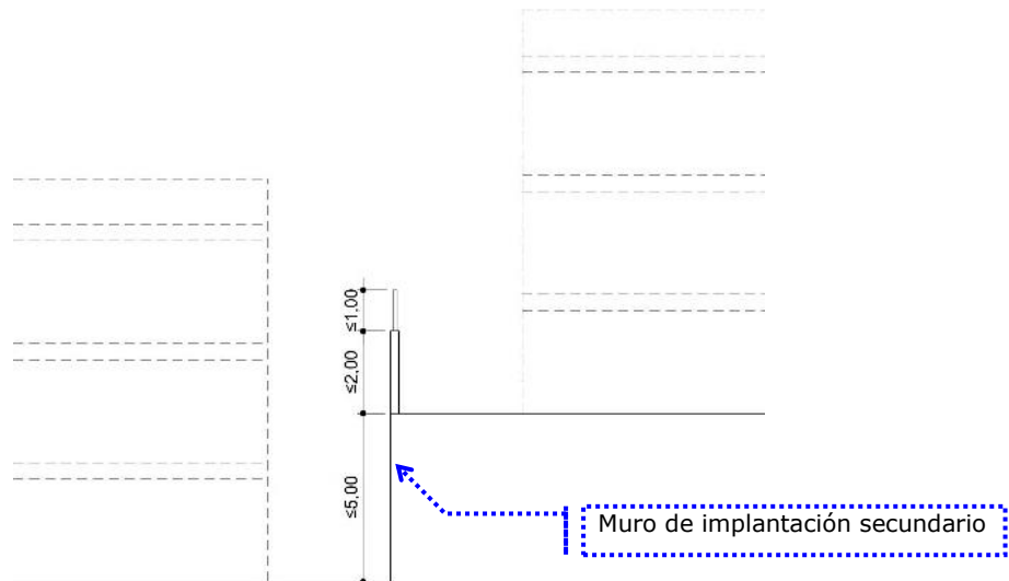
Muros de contención de espacios libres con colindantes y altura de cerramientos
