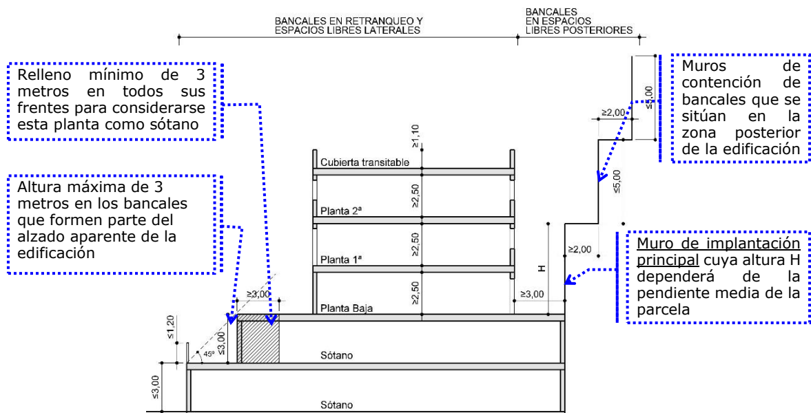
Ejemplo de dimensiones de muros y bancales en una parcela ladera arriba
