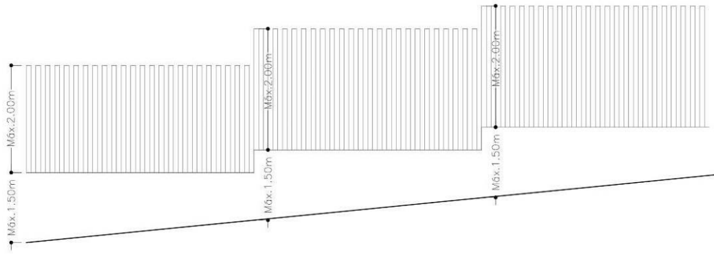
Cerramiento escalonado con frente a vía con pendiente
