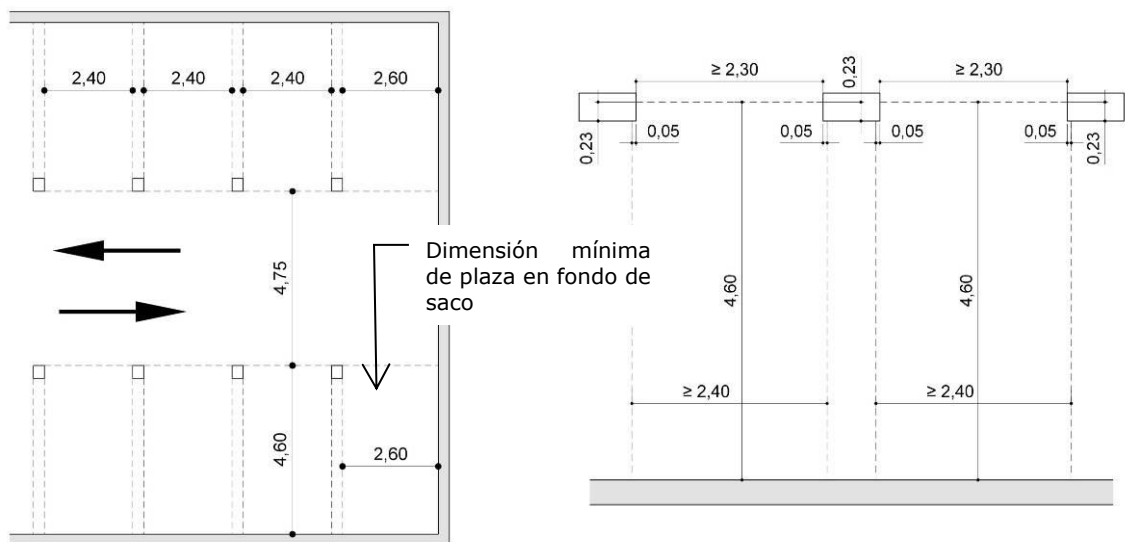
Dimensiones con reducción por existencia de pilares o similares
