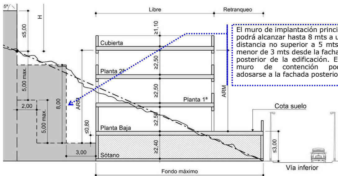
Parcelas ladera arriba con pendientes entre el 35% y el 50%
