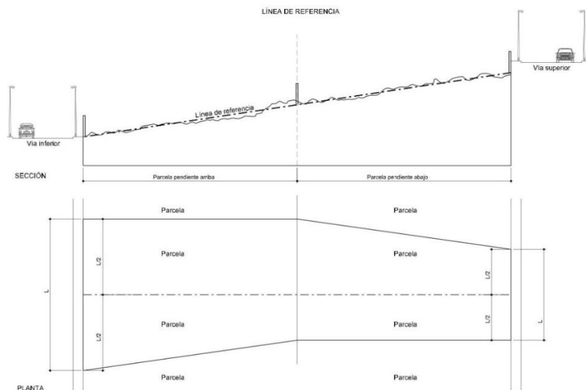
Ejemplo de trazado de línea virtual de referencia
