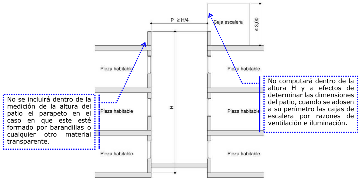
Condiciones del patio de parcela cerrada
