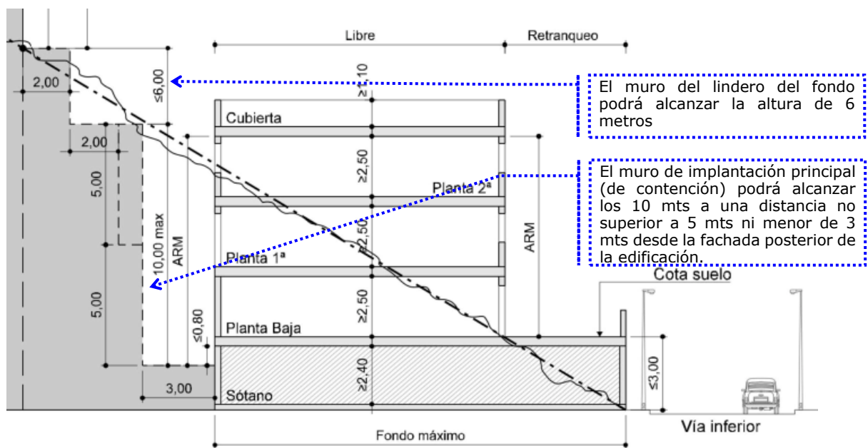
Parcelas ladera arriba con pendientes superiores al 50%
