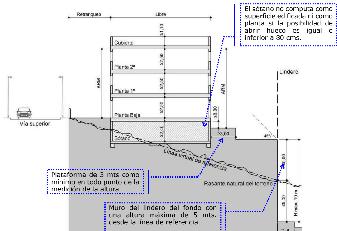
Sección característica ladera abajo con pendientes entre el 15% y el 35%
