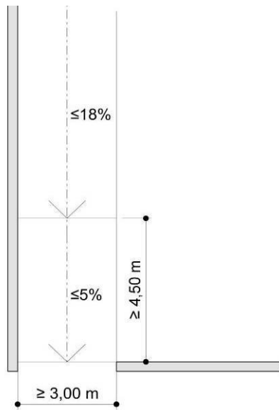
Acceso recto con sentido alternativo
