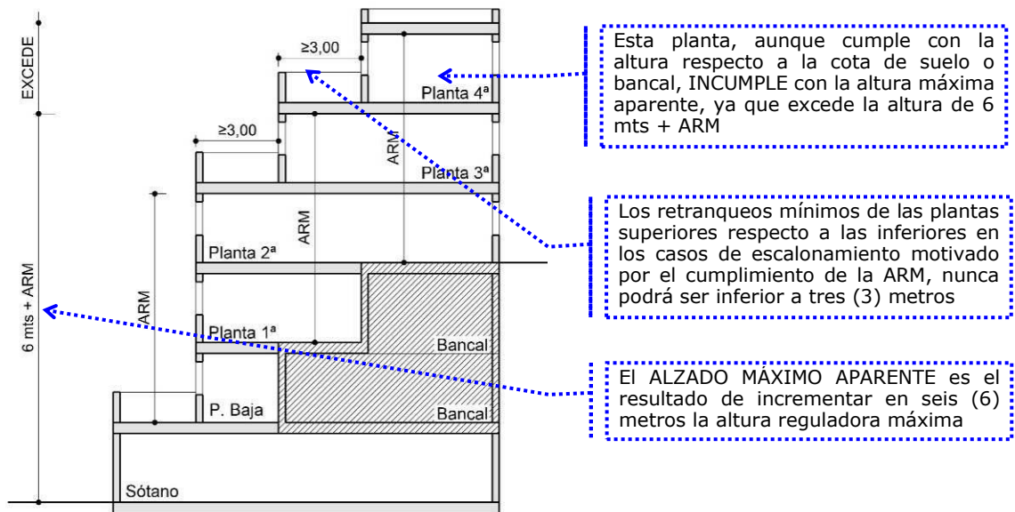
Ejemplo altura máxima aparente para una edificación ladera arriba con tres (3) plantas de altura máxima
